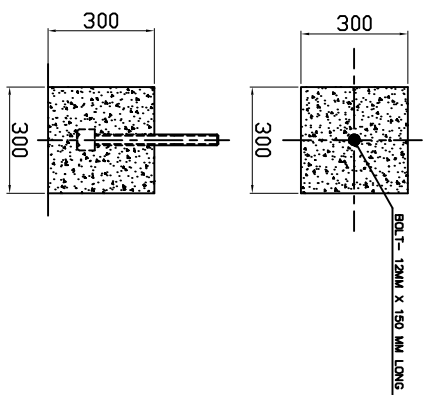
DET. OF MKD. - "X"
