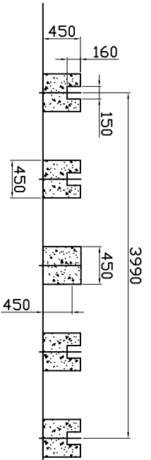
ELEVATION
